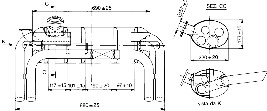
COMPLESSIVO SCHEMATICO DEL DISPOSITIVO SILENZIATORE DI SCARICO
